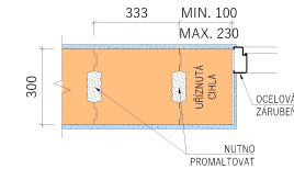
- VAZBA U DVEŘNÍHO OSTĚNÍ, 2. ŘADA ZDIVA
