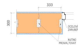
- VAZBA U DVEŘNÍHO OSTĚNÍ, 1. ŘADA ZDIVA
